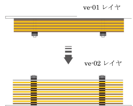
Figure 1 ve-02 構成図
