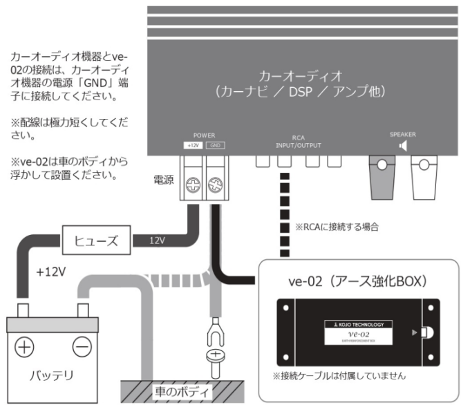
Figure 7 ve-02 の接続方法
