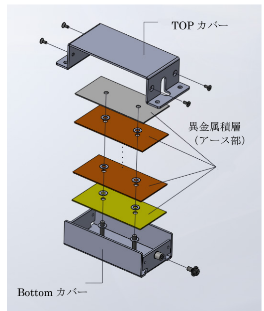
Figure 1 ve-02 構成図
